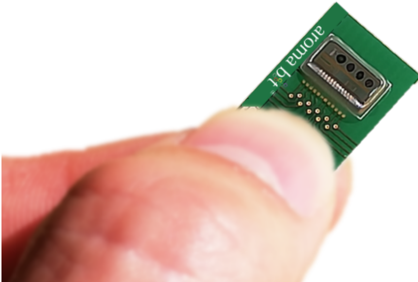
新販売のシリコン CMOS ニオイセンサー開発キット (品名：5C-SSM)
